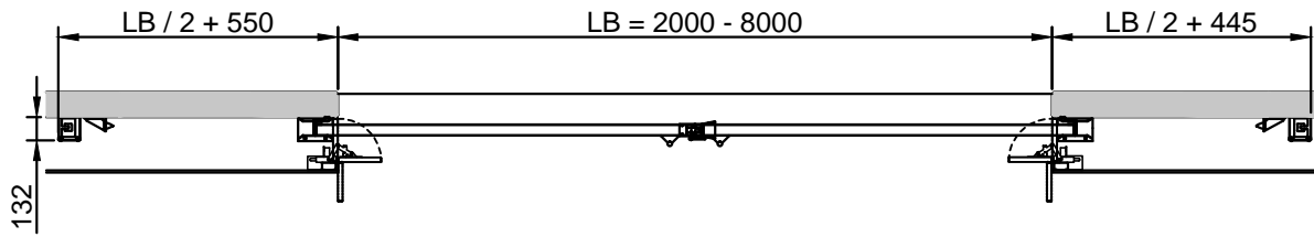
Horizontalschnitt
