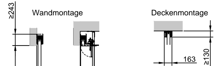
Vertikalschnitt
