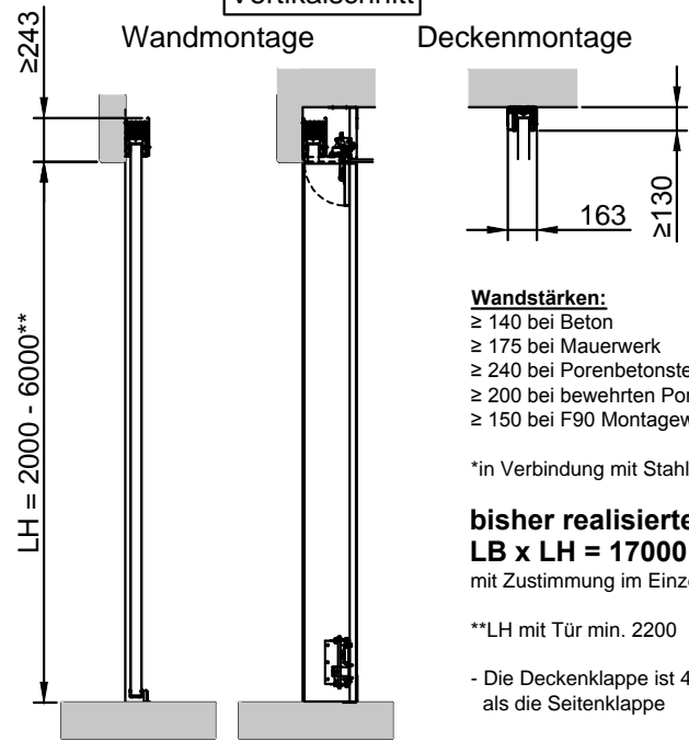
Vertikalschnitt
