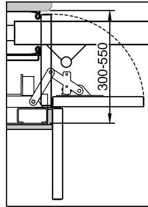
Seitenklappe "optional"
