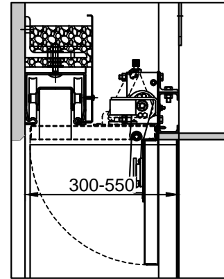
Deckenklappe "optional"
