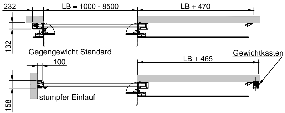
Horizontalschnitt
