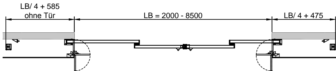
Horizontalschnitt
