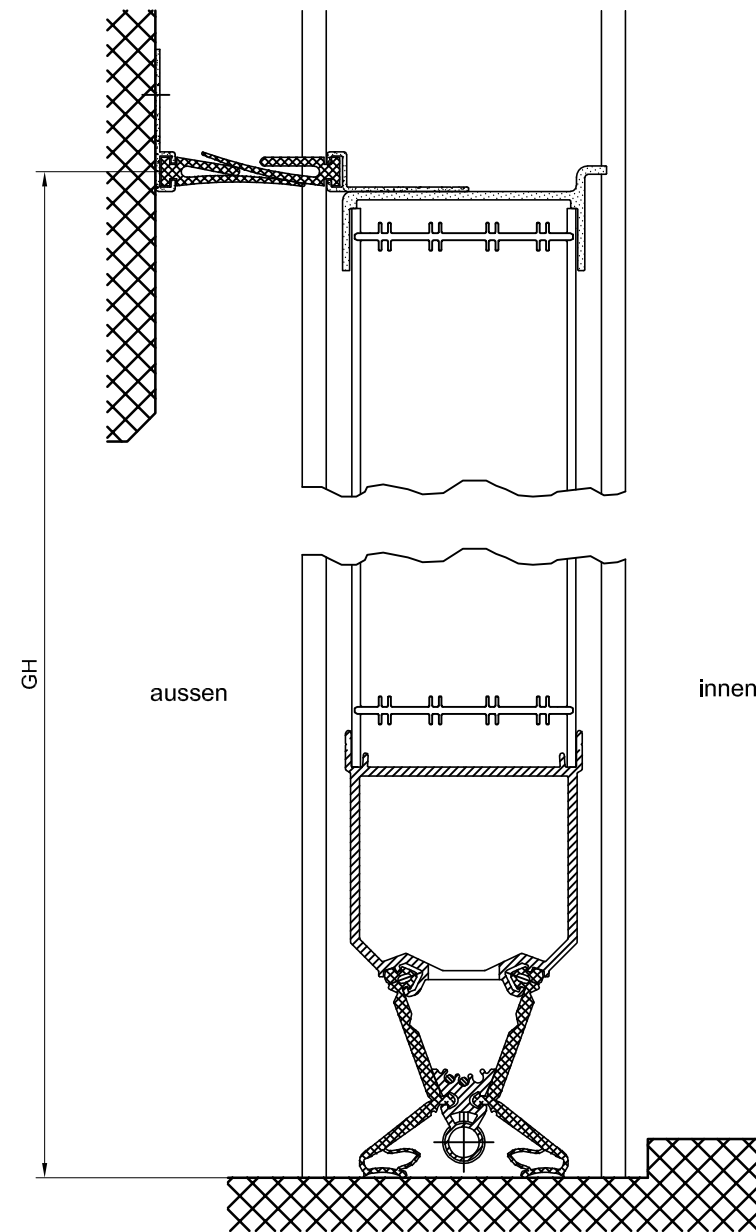
Vertikalschnitt
