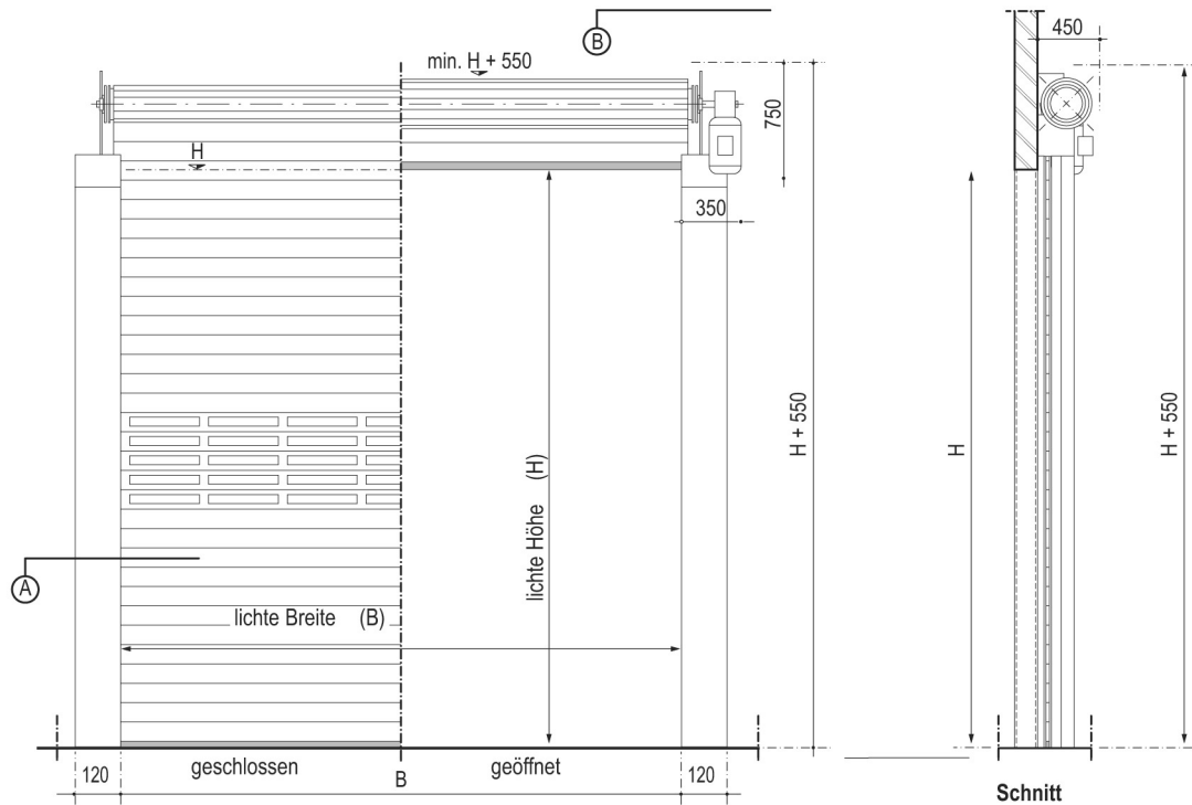
Vorderansicht
